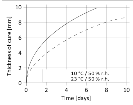
แผนภาพที่ 1: อัตราการแห้งตัวของ Sikaflex®-291
